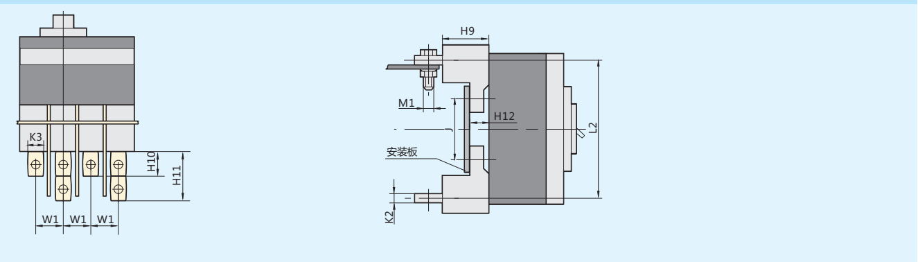
插入式接线图(安装尺寸见表14)
