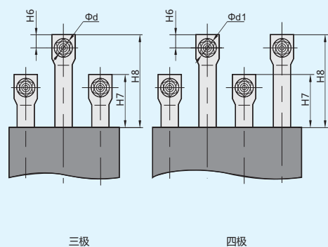
板后接线开孔图(尺寸见表14)
