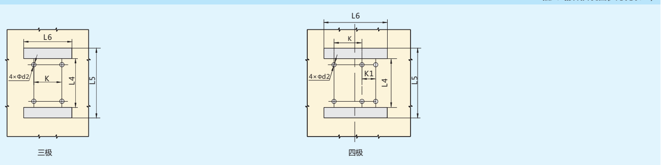
插入式接线开孔图(尺寸见表14)
