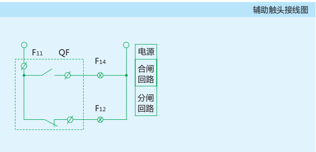
辅助触头接线图
