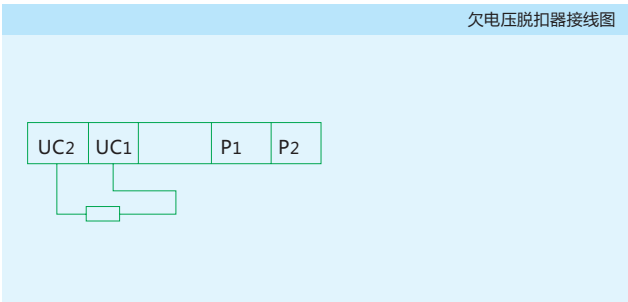
欠电压脱扣器接线图
