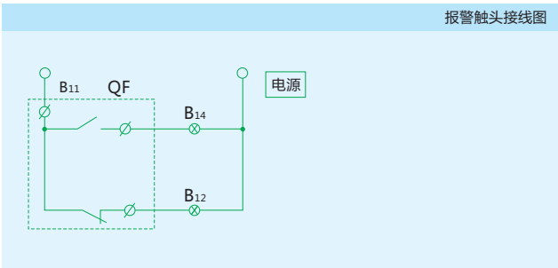
报警触头接线图
